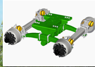
Roll-Over bogie met naloopas
