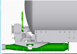
Wormpomp met stenenvanger en voorafuitrusting voor front-Jumbo
